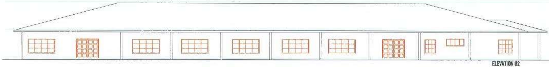
ELEVATION 02
