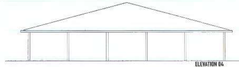
ELEVATION 04
